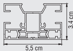
Doppelführungsschiene
