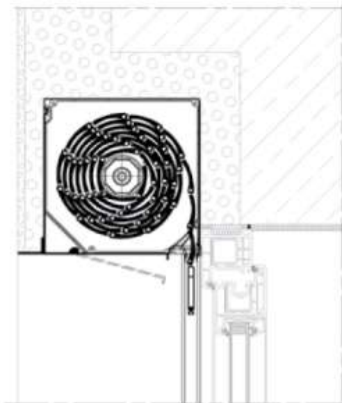
SP – Rollläden
