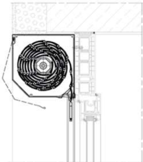
SK – Rollläden
