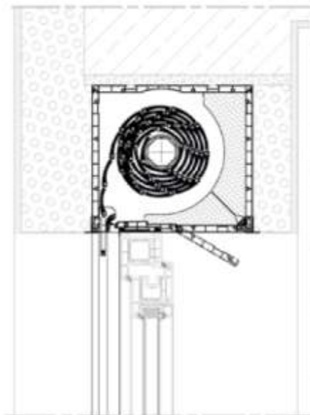
SKT – Rollläden
